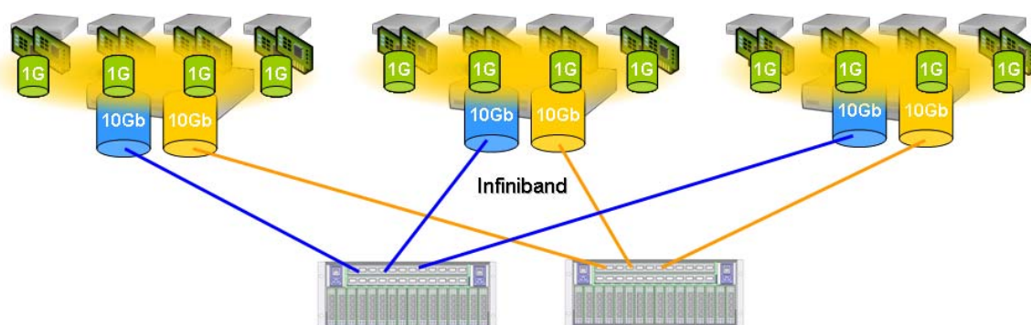
図：仮想サーバ環境下での接続概念図
