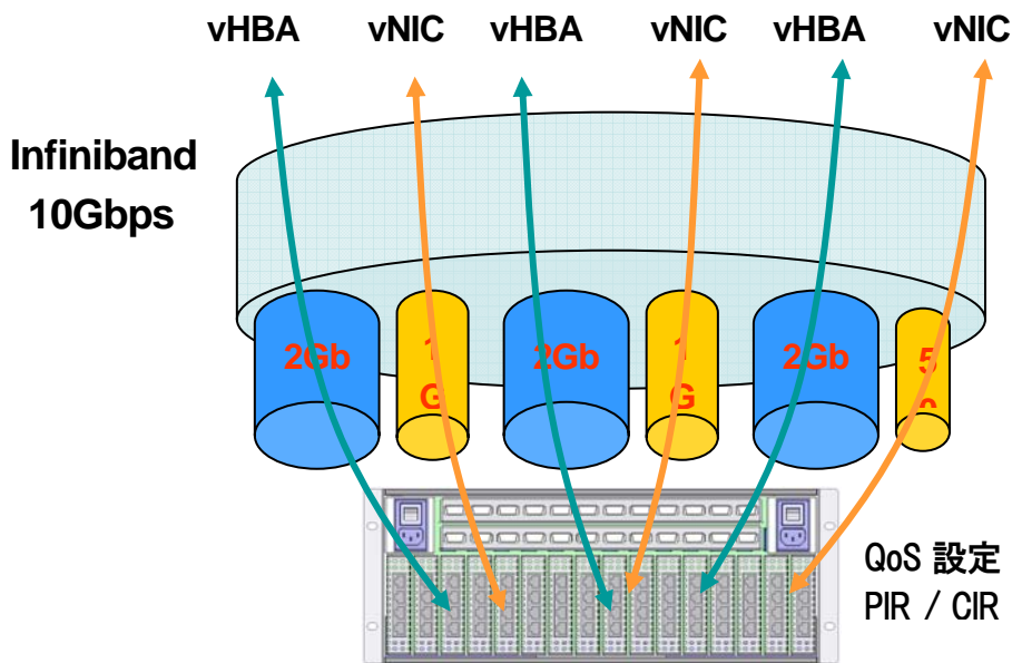
図:I/O 仮想化概念図
